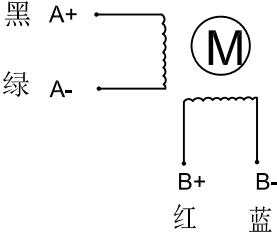
接线方式
